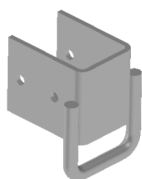
Suporte de Amarração de Carga 21.00.018
