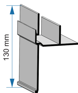
Saia 130 50.01.001
