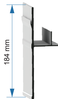
Saia 184 50.04.003
