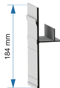
Saia FC 184 50.04.003
