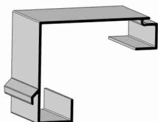
Coluna 50.05.020
