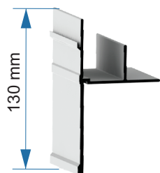
Saia 130 50.07.001
