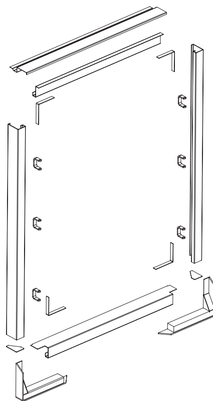
Quadro Traseiro
