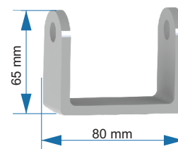
Cavalete Reto 10.02.010
