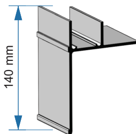
Saia 140 50.02.002
