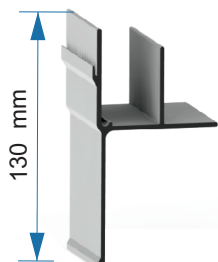
Saia 130 50.01.002
