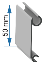
Perfil Intermediario 99.00.417
