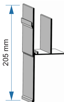
Saia 205 mm 50.01.005
