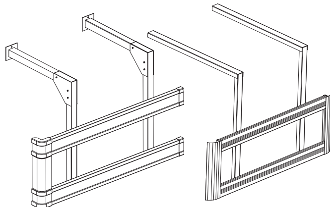
Protetor de ciclista
