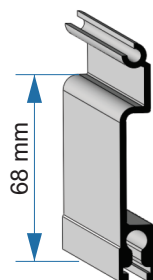
Perfil Inferior 99.00.123
