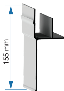
Saia Nova 155 50.01.004
