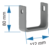
Cavalete largo Tras. Ant. 99.00.172
