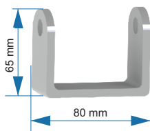
Cavalete Reto 10.02.010
