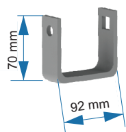
Cavalete Tras. 10.04.011
