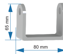
Cavalete Reto 10.02.010
