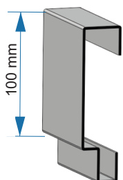
Coluna Q. Lat. 100 mm 99.00.027
